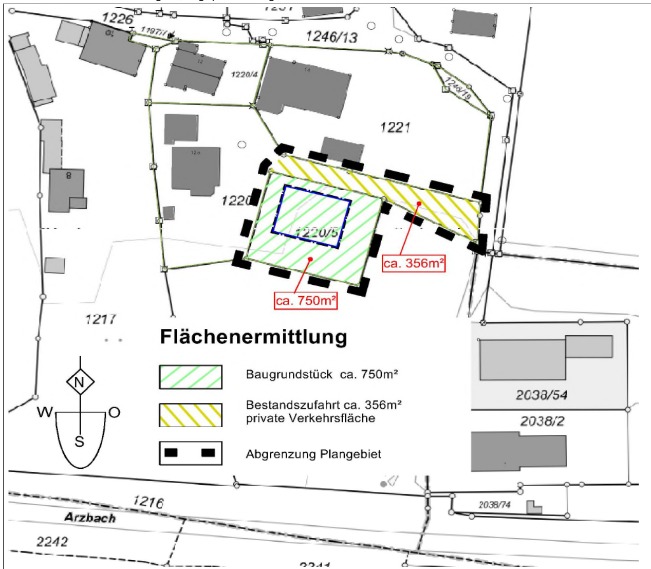
Abb. 2: Flächenermittlung
